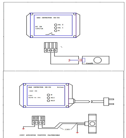
Signalizatoriaus ir vožtuvo sujungimo schema
